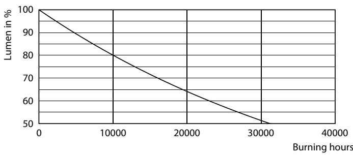
Lumen Maintenance Diagram - 11A19/CNG/850/FR/P/E26/D 12/1CT
