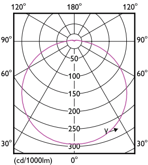
Light Distribution Diagram - 26UFO/PER/830/FR/P/E26/ND 4/1PF
