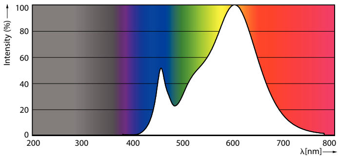
Spectral Power Distribution Colour - 26UFO/PER/830/FR/P/E26/ND 4/1PF
