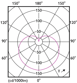
Light Distribution Diagram - 8.8A19/PER/927/FR/P/E26/D2D/T20 4/1PF
