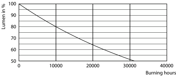
Lumen Maintenance Diagram - 2.3BA11/PER/UD/CL/G/E12/WGD 6/3PFT20
