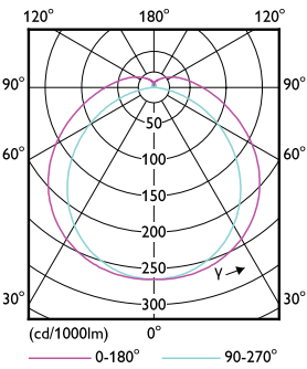
LEDtube MAS 8,9W G13 1500lm
