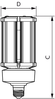
36CC/LED/840/ND E26 G2 BB 6/1
