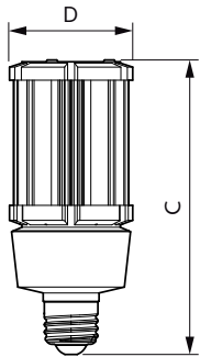
18CC/LED/850/ND E26 G2 BB 6/1
