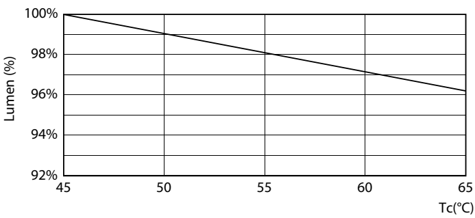
LEDtube_70K_1_LumenVsTc-LMP
