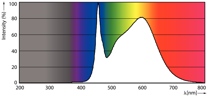
LEDtube_G13_840-POC
