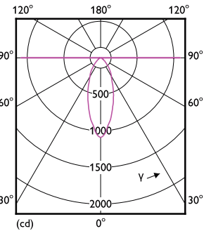
LEDspots MAS G1 8W PAR30L E26 930 40D
