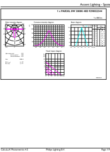
LEDspots MAS G1 8W PAR30L E26 930 40D
