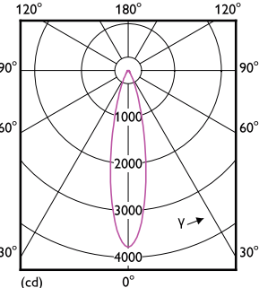
LEDspots 10W PAR38 E26 930 25D
