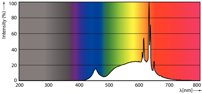
LEDspots 10W PAR38 E26 930 25D
