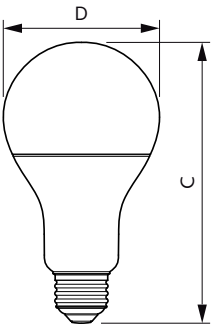
A21 120V 12.2-75W 1100lm 3000K E26 D
