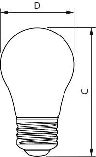
A15 120V 40W 450lm 5000K E26 D CL
