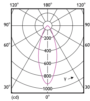
LEDspot E26 PAR20
