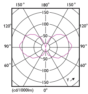
LEDbulb BA11 4,5W E12 820 Amber
