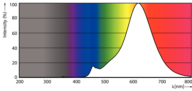
LEDbulb 4,5W BA11 E12 820 Amber
