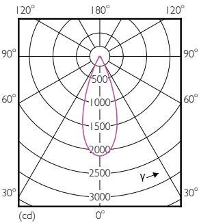
LEDspot E26 40°
