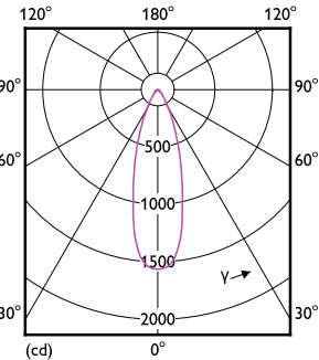
LEDSpot PAR20 E26 4000K 40D
