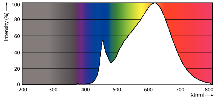
LEDspot E26
