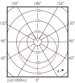
60W E26 A19 FR 250D 927 2700K
