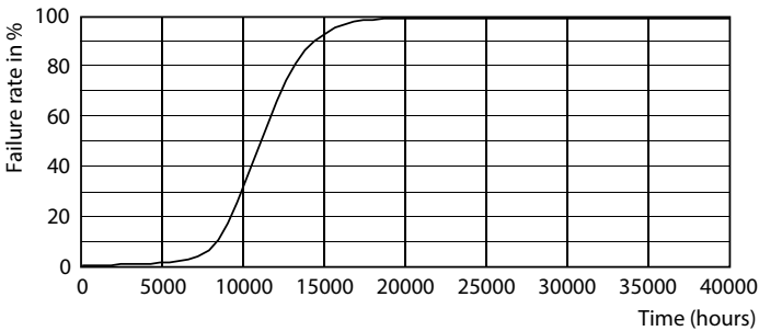
60W E26 A19 FR
