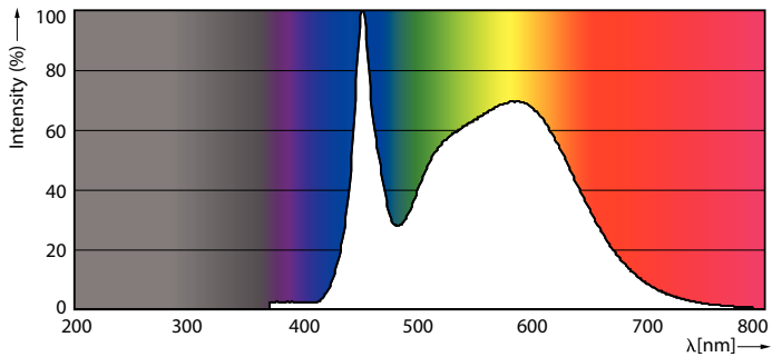
60W E26 A19 FR
