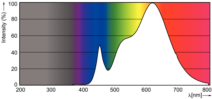
11-50W AR111 /930
