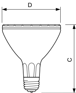
CDM-R Elite 35W/930 E26 PAR30L 10D
